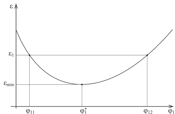
Рис. 1. Зависимость угла отклонения луча \varepsilon от угла падения \varphi_1 на грань призмы
